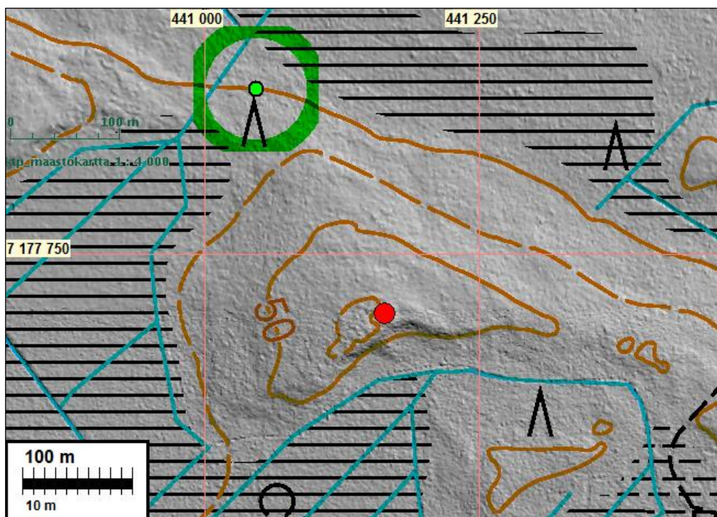
Rakenne punaisen pallon kohdalla. Kivetön alue ei erotu maastomallissa
