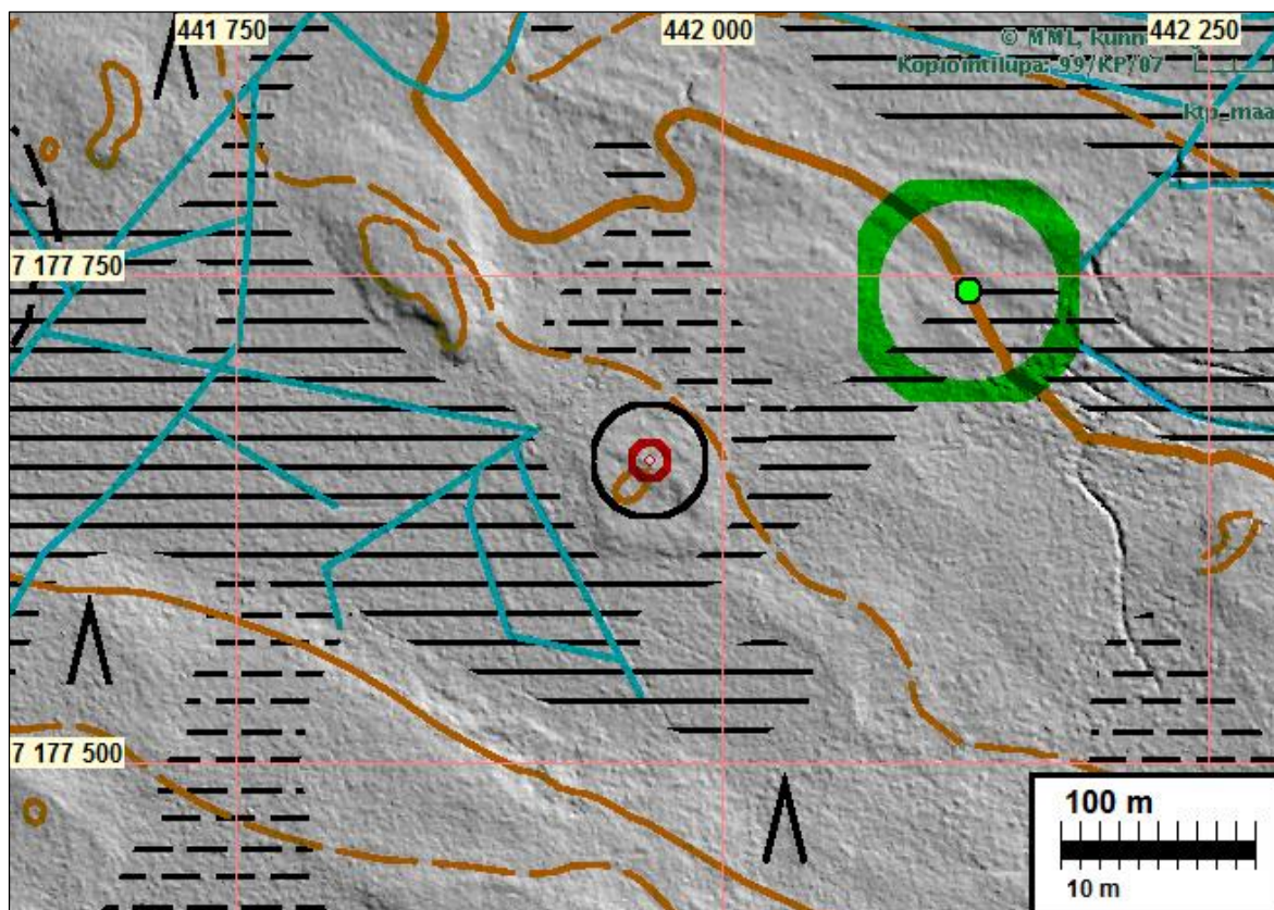
Kuoppa sijaitsee punaisen ympyrän sisällä. Voimalapaikka vihreällä
