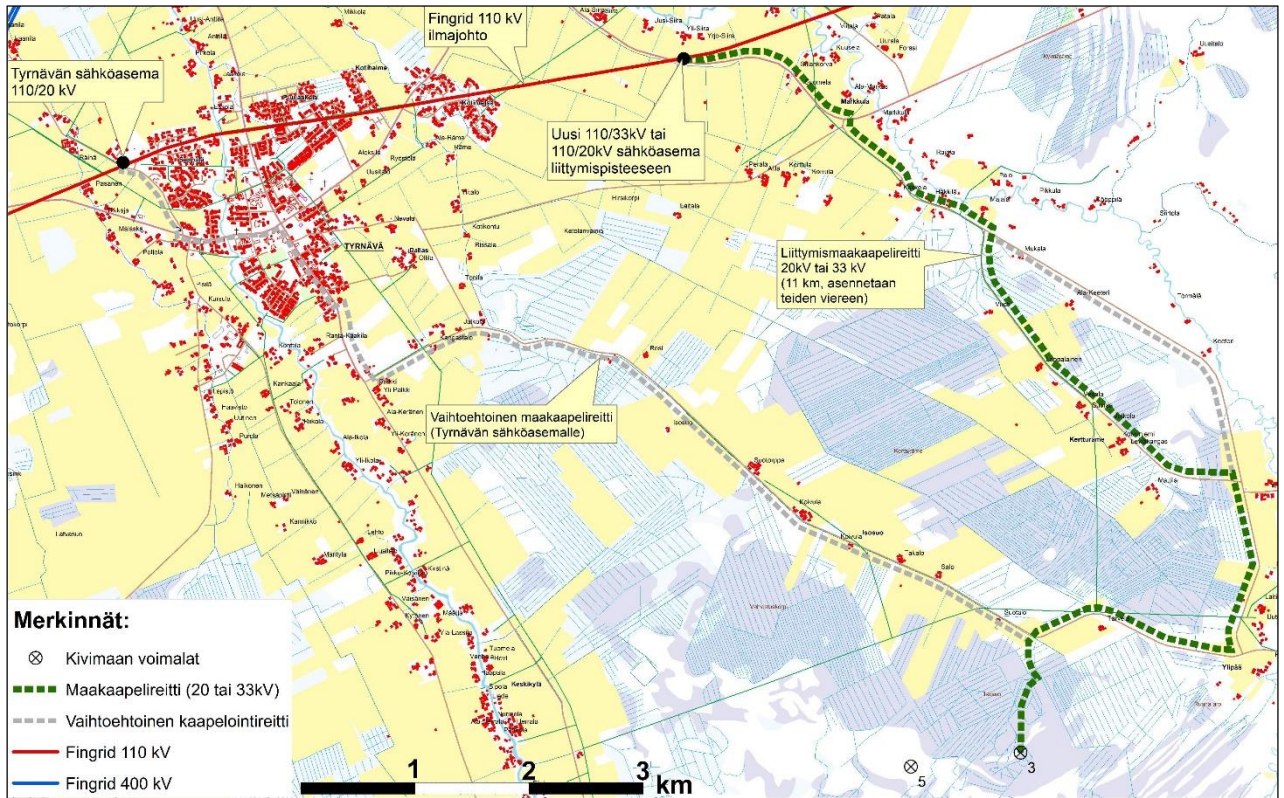
Vaihtoehtoiset sähkönsiirtomaakaapelireitit tuulipuiston pohjoispuolella
