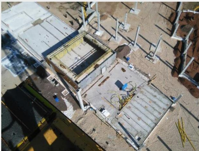
VSS: n ja keittiön välinen, valettu, paalulaatta
